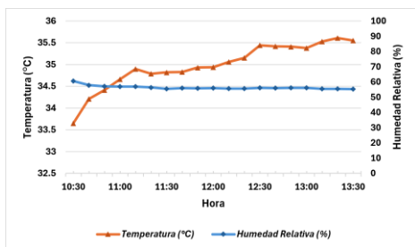
Figura 9. Temperatura y humedad relativa en residencia de Santiago con sistema Zinc + Foam.
