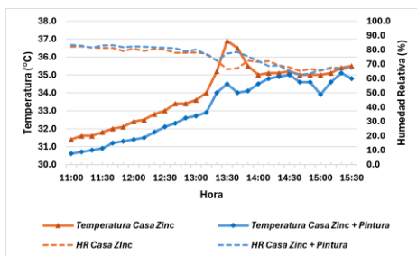
Figura 13. Comparación de temperatura y humedad relativa entre Casa A y Casa B con techo de zinc sin tratamiento y techo con pintura termoaislante, respectivamente. Periodo 11:00 A 15:30.
