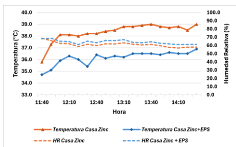
Figura 12. Comparación de temperatura y humedad relativa entre Casa A y Casa B con techo de zinc sin tratamiento y techo con zinc más núcleo de EPS, respectivamente. Periodo 11:40 A 14:30.
